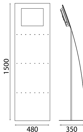
Verkaufsständer für LCD-Anzeige 15"
